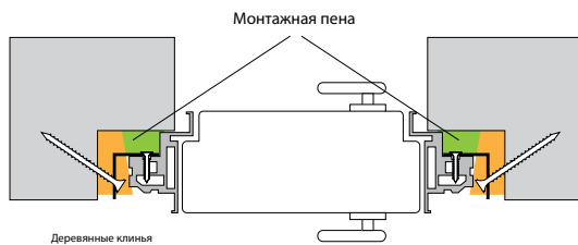
Заполнить полости монтажной пеной
