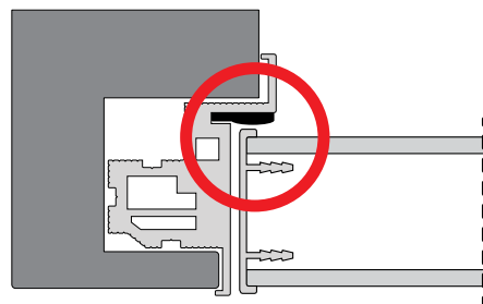
Вариант отделки под торцевой профиль
