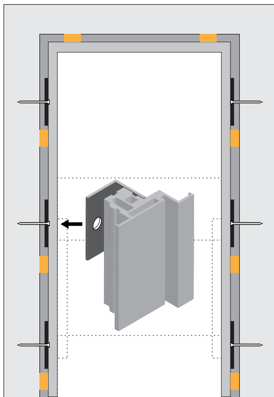
Зафиксировать раму в проеме при помощи саморезов.
