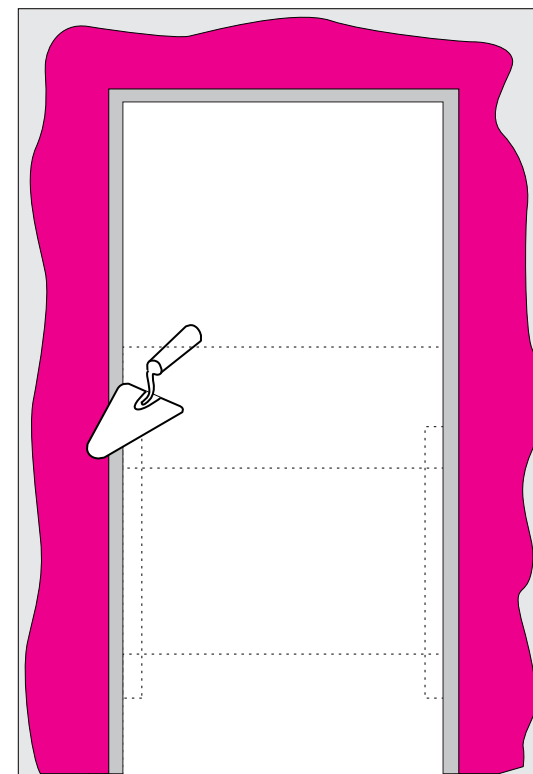
Через 24 часа удалить излишки монтажной пены. Зашпатлевать зазоры.
