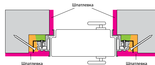
Через 24 часа удалить излишки монтажной пены. Зашпатлевать зазоры.
