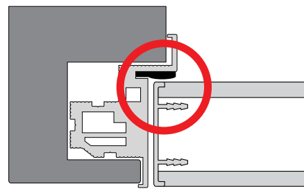
Вариант отделки в одну плоскость с торцевым профилем
